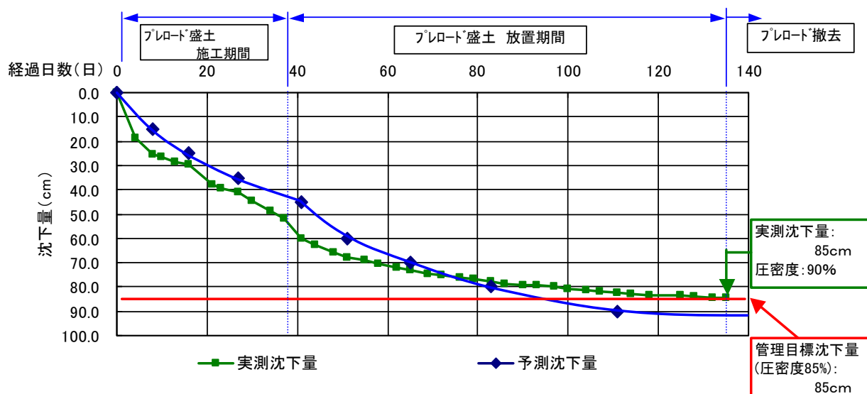
< 沈下曲線 >
