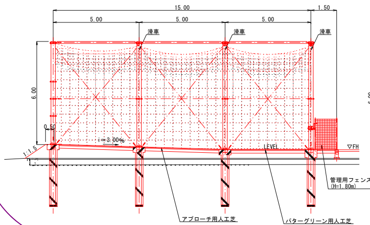
側面図
